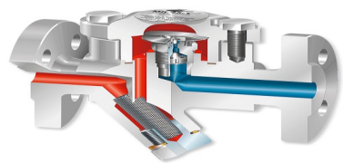
PURGEURS DE CONDENSATS
